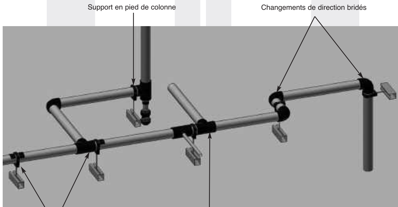
Point fixe avec demi coquille (réf. HPTF)
